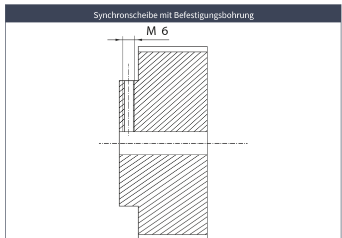
Gewinde-Bohrung M6 mittig Nabe
