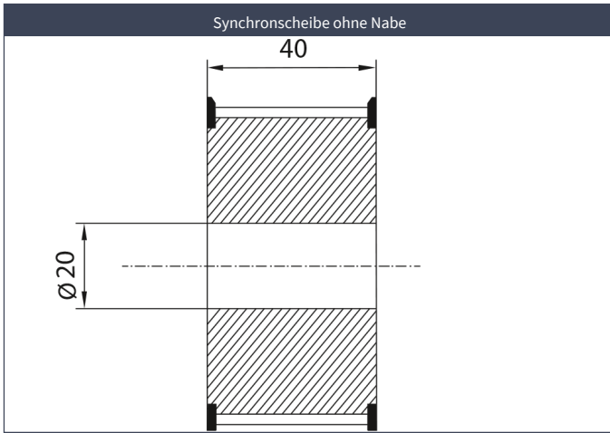
Synchrone Scheibe Al 40 AT10/24-2 d=20 H7
