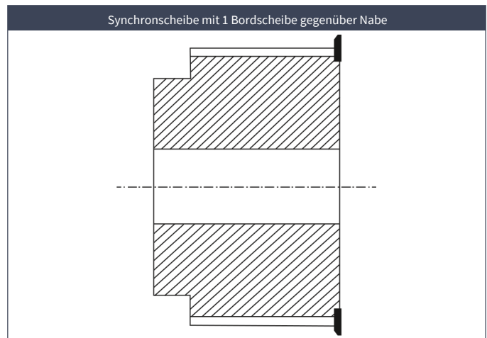
1 Bordscheibe gegenüber Nabenseite: -1g
