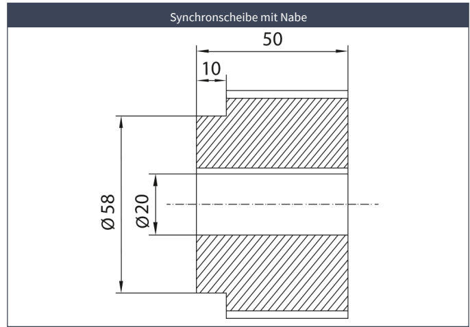
Synchrone Scheibe Al 50 AT10/24-0 Nabe \varnothing 58 \times 10 d=20 H7 mit Nut
